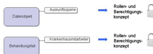
Datenmodell (Tz. 1.10/1.11)
