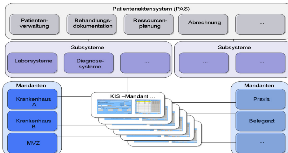
Krankenhausinformationssystem (KIS)
