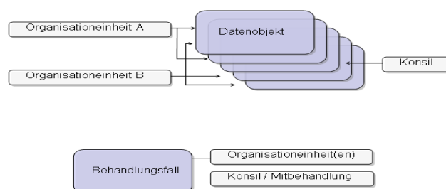
Datenmodell (Tz. 1.4)
